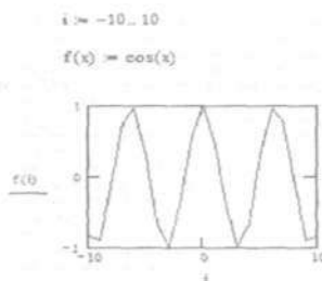
11.13-rasm. \cos(x) grafigi.
