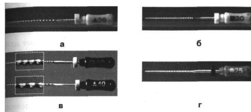
Рис. 10.15. Инструменты для препарирования корневого канала: а — K-Reamer — инструмент для прохождения корневого канала; б — K-File — инструмент для расширения корневого канала; в — различие в шаге режущей части файла и римера; г — Hedstrom — (бурав Хедстрема) — инструмент для выравнивания стенок корневого канала.
