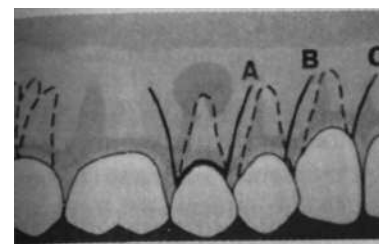
Рис. 10.41. При наличии искусственных коронок можно проводить разрез по траектории A, B или C. Схема.
