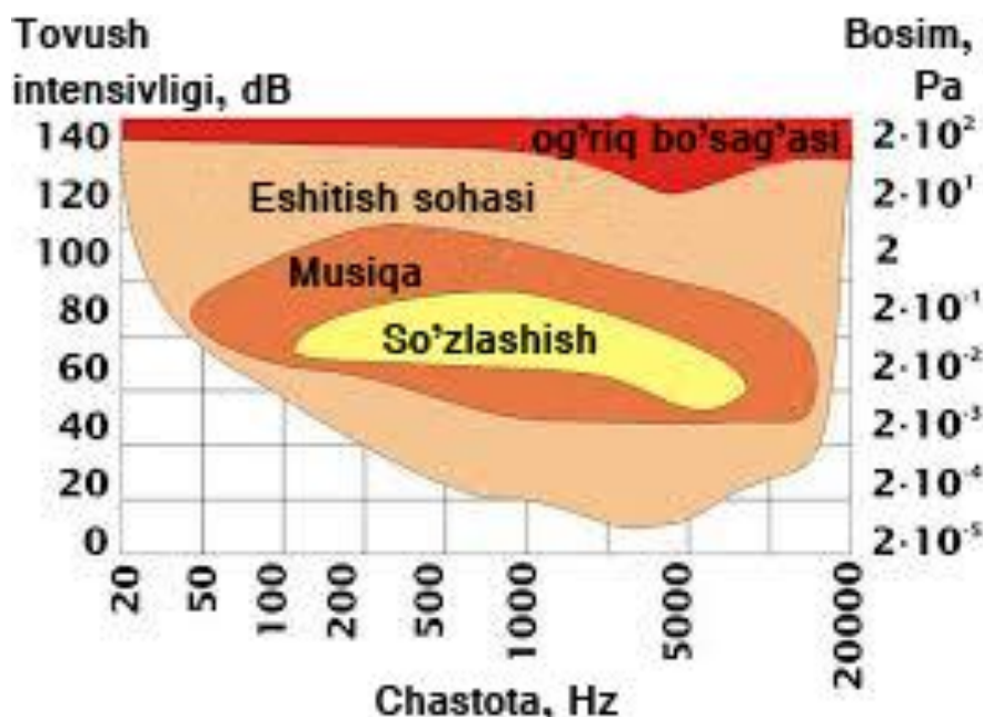
5.8-rasm. Odam qulog'i eshitish va og'riq bo'sag'alari
