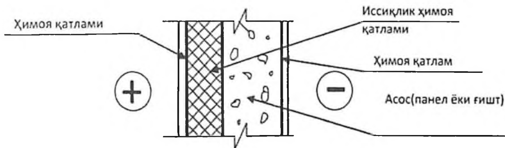
1-расм. Ички томондан иситиладиган девор қурилмаси.
