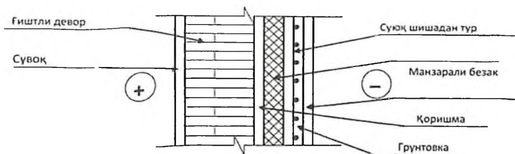
3-расм. Ҳўл турдаги иситиш тизими қурилмаси.
