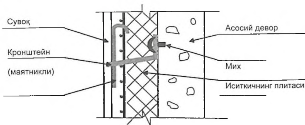
4-расм. Силжувчан кронштейнларнинг маҳкамланиш тизими. («термофасад тизими»).
