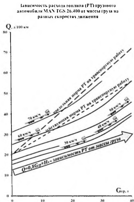
Рисунок 2. Зависимость расхода топлива (РТ) грузового автомобиля MAN TGS 26.400 от массы груза на разных скоростях движения.
