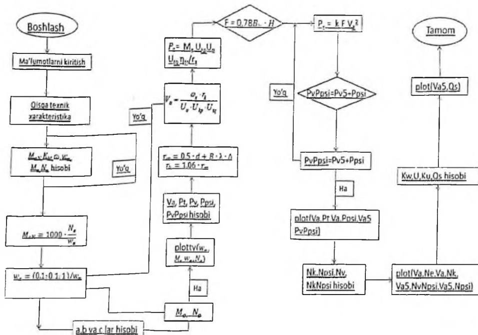
1-расм. Берилган йўл шароитида юк автомобилнинг ёнилғи сарфини аниқлаш алгоритми.
