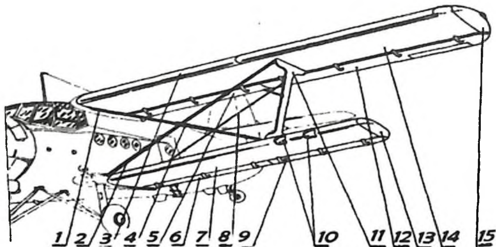
Рис.1. Бипланная коробка.
