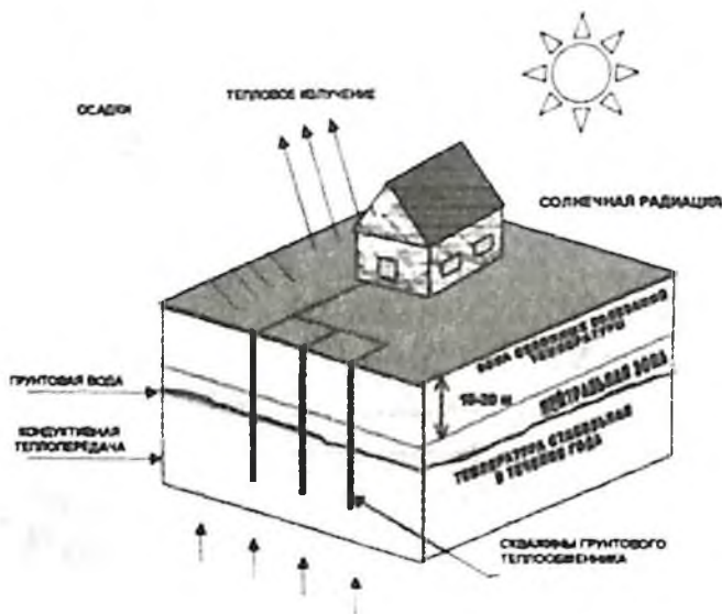
Рис. 1. Факторы, формирующие температурный режим грунтового массива системы сбора низкопотенциальной теплоты поверхностных слоев Земли.
