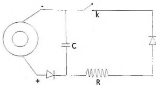
3-расм. Зарядловчи пойафзалнинг схемаси.
