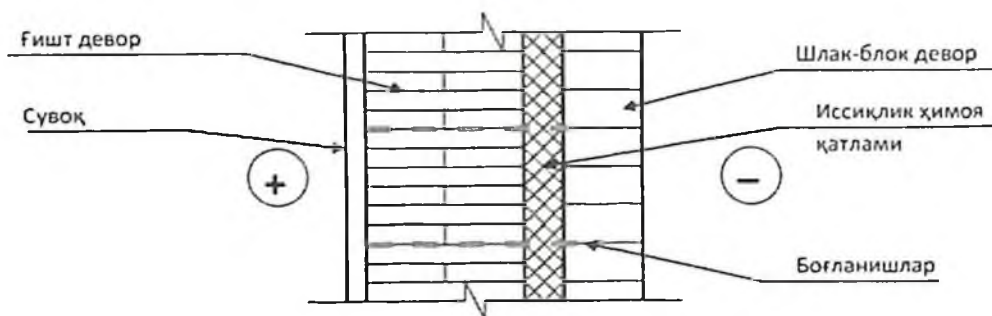
2-расм. Ташқи томондан ғишт қопланган қўп қатламли юк кўта- рувчи ташқи девор қурилмаси.
