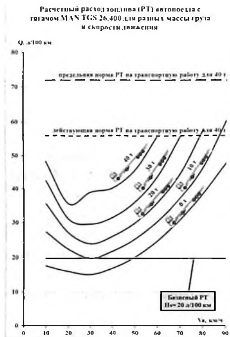
Рисунок 1. Расчетный расход топлива (РТ) грузового автомобиля MAN TGS 26.400 для разной массы и скорости движения.
