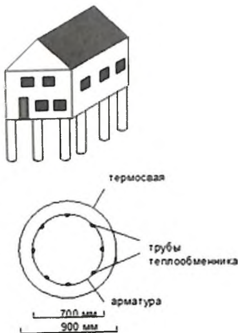
Рис. 5. Схема грунтовых теплообменников, замоноличенных в фундаментные сваи термосваи, и поперечное сечение термосвай
