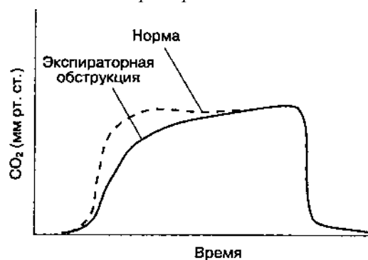
Рис. 23-1. Капнография при экспираторной обструкции дыхательных путей
