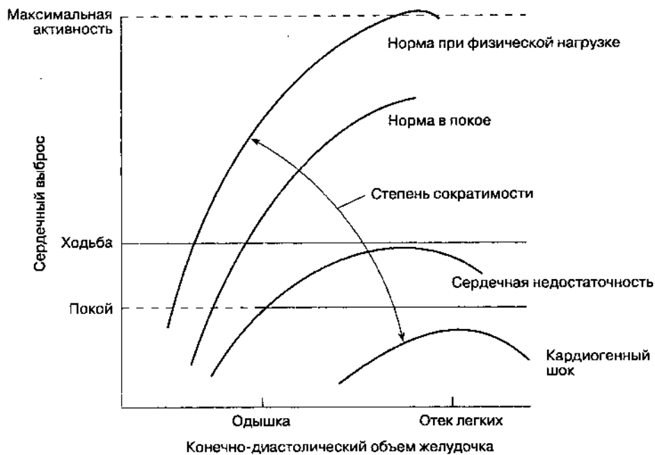
Рис. 19-5. Закон Старлинга
