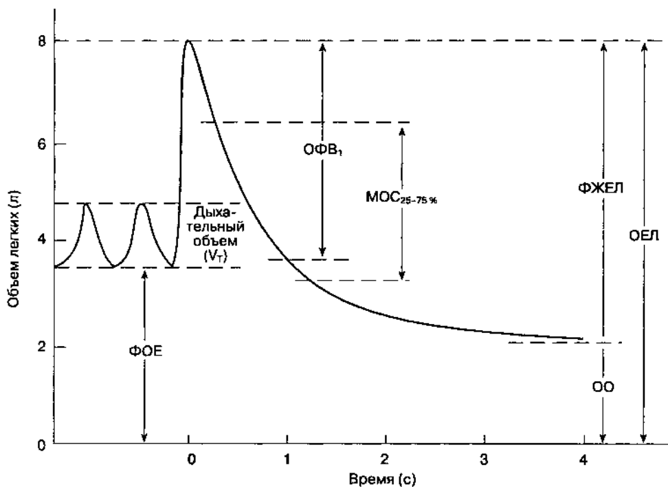
Рис. 22-10. Кривая форсированного выдоха у здорового человека. Скорость форсированного выдоха ( ОФВ_{25-75\%} ), также называется максимальной скоростью потока в середине выдоха ( МОС_{25-75\%} )
