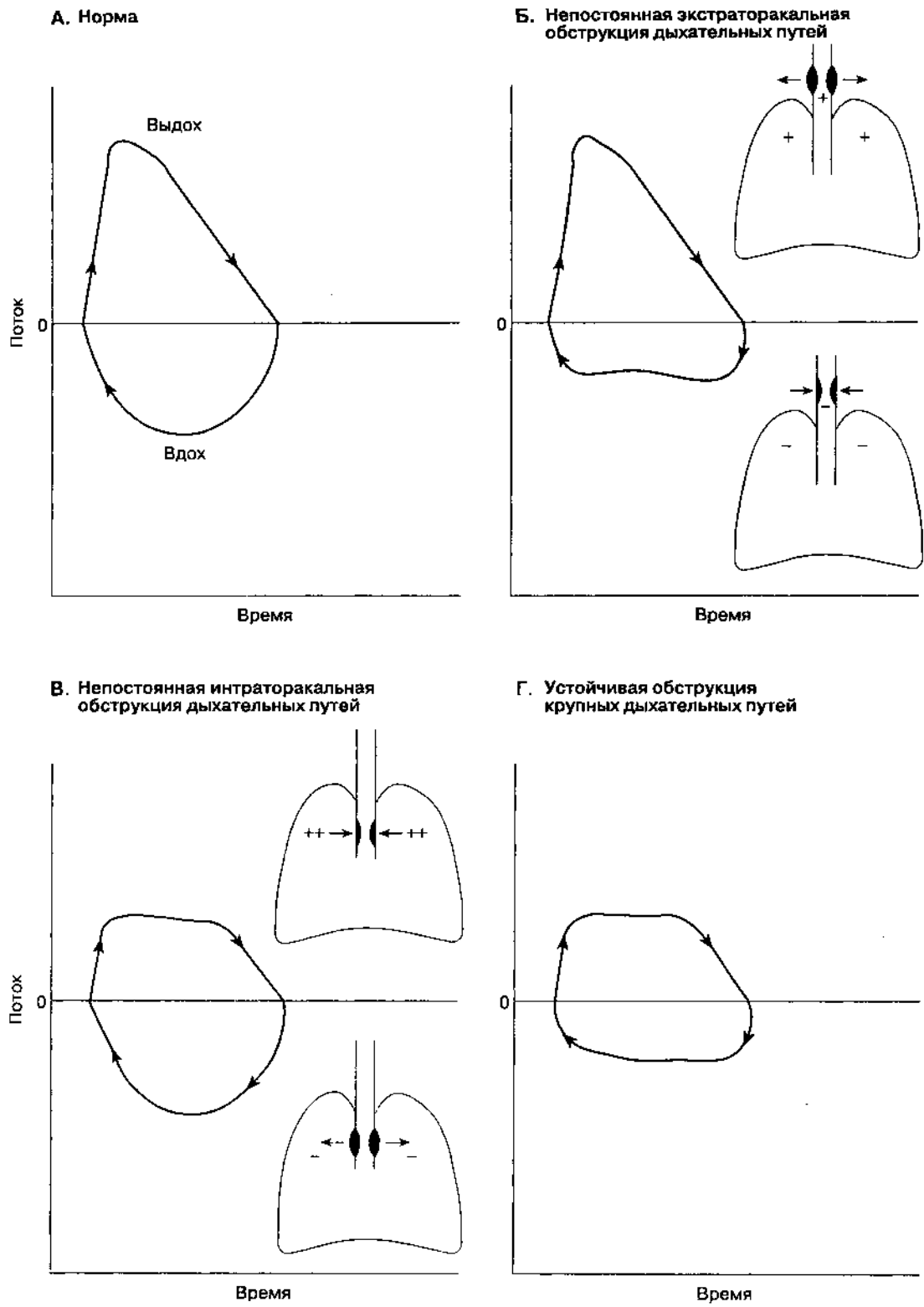
Рис. 24-10. Петли "поток-объем"
