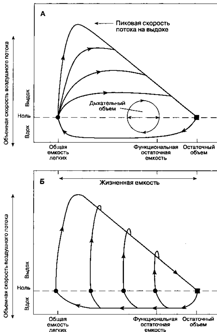
Рис. 22-9. Поток газа (А) при форсированном выдохе после максимального вдоха с различным усилием и (Б) с максимальным усилием после вдохов различной глубины. Отметим, что окончательный поток выдоха не зависит от усилий дыхательных мышц при любом исходном объеме легких. (С разрешения. Из: Nunn J. F. Applied Respiratory Physiology , 3rd ed. Butterworths, 1987.)
