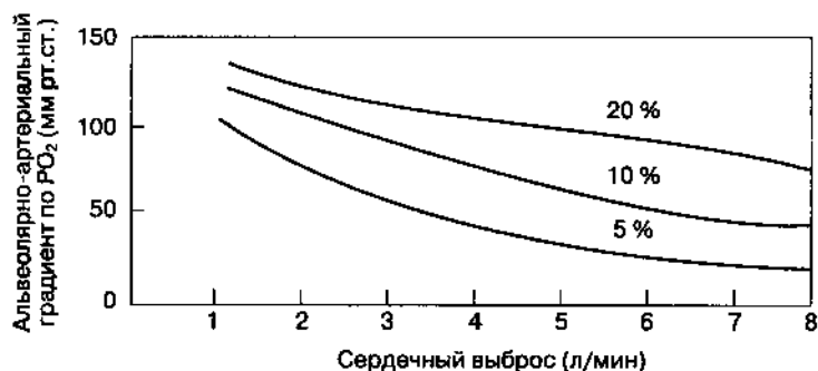
Рис. 22-20. Влияние сердечного выброса на альвеоларно-артериальный градиент по PO_2 при различной степени шунтирования ( \dot{V}O_2 = 200 мл/мин и P_{iO_2} = 180 мм рт. ст.). (С разрешения. Из: Nunn J. F. Applied Respiratory Physiology, 3rd ed. Butterworths, 1987.)
