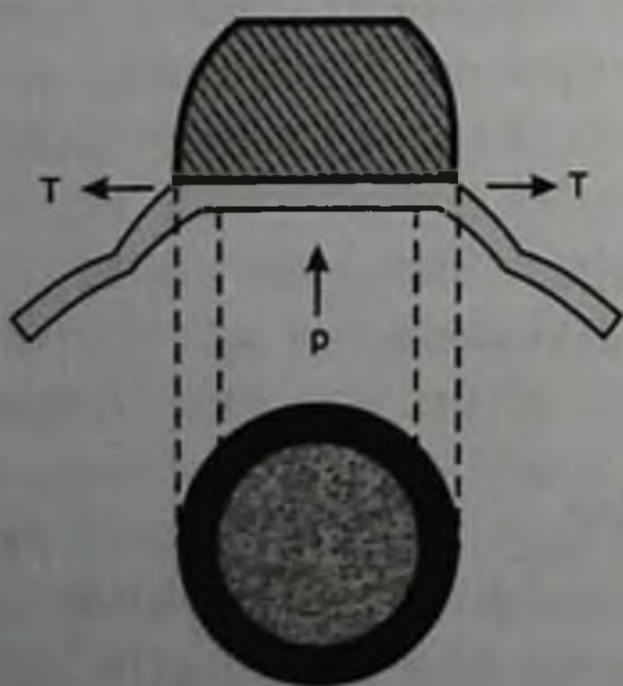
Рис. 4.6. Сплющивание роговицы площадкой тонометра Маклакова
