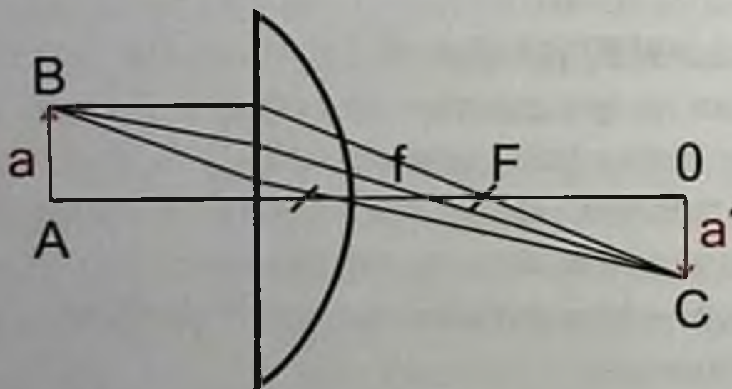
Рис. 5.3. Формирование изображения собирающей сферической линзой: a — рассматриваемый предмет; a' — изображение предмета; АО — оптическая ось; F — главный фокус; F' — один из фокусов, образованный собирающимися лучами, идущими от предмета; BC — лучи, проходящие через главную точку линзы
