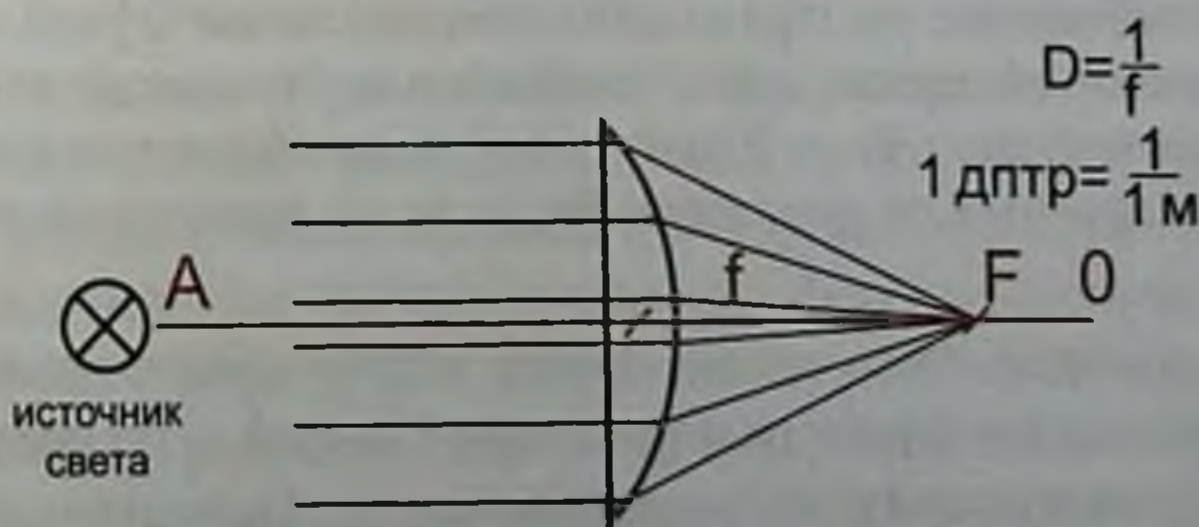
Рис. 5.1. Строение и действие плосковыпуклой сферической линзы: AO — оптическая ось; F — главный фокус; f — главное фокусное расстояние; D — преломляющая сила линзы
