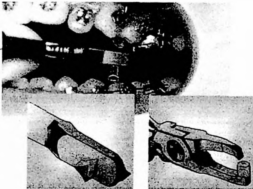
Рис. 91 Инструменты для работы с ортодонтическими кольцами: кольцевой адаптер (а,б) и специальные щипцы (в).
