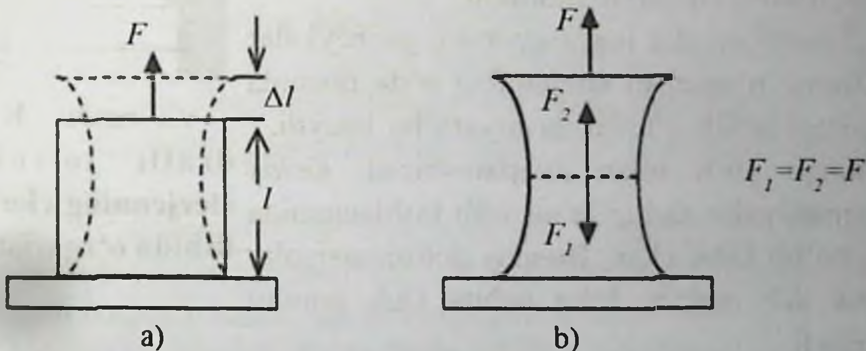
1.1.-rasm. Cho'zilish deformatsiyasi (a); cho'zilishda yuzaga keluvchi kuchlar (b)
