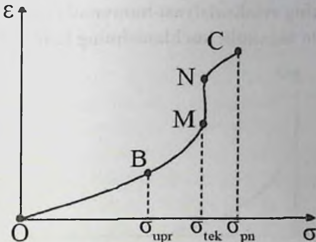
1.7-rasm. Deformatsiyaning kuchlanishga bog'liqligi cho'zilish diagrammasi.
