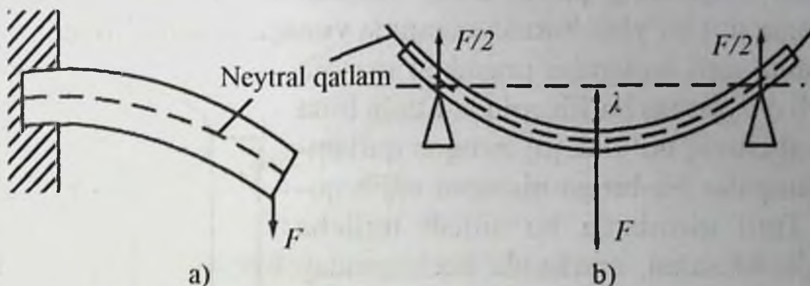
1.5-rasm. Egilish deformatsiyasi.
