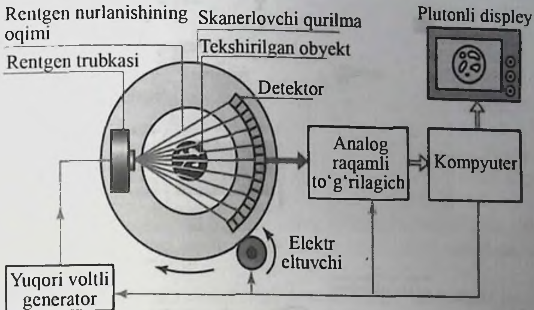
8.7-rasm. Kompyuter tomografining prinsipial sxemasi
