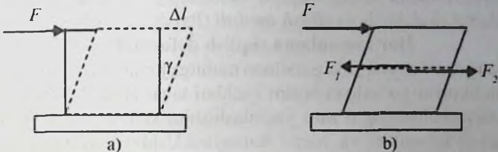
1.3-rasm. Siljish deformatsiyasi (a); siljishda yuzaga keluvchi kuchlar (b)
