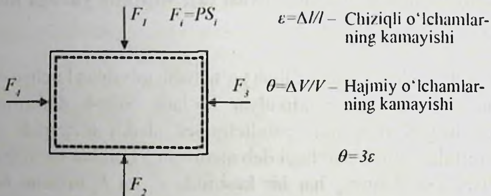
1.4-rasm. Har tomonlama (gidrostatik) siqilish.
