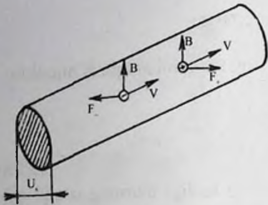
3.16-rasm. Magnit maydoni tomonidan turli xil ishorali zaryadga ta'sir etuvchi kuchlar
