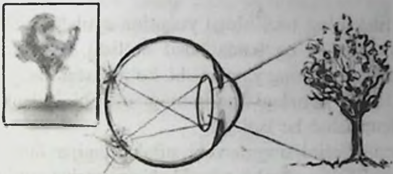
7.19-rasm. Astigmatik ko'zda tasvirning ko'rinishi (daraxt tasviri bir necha marta fokuslanib, xira tasvir hosil bo'ladi)
