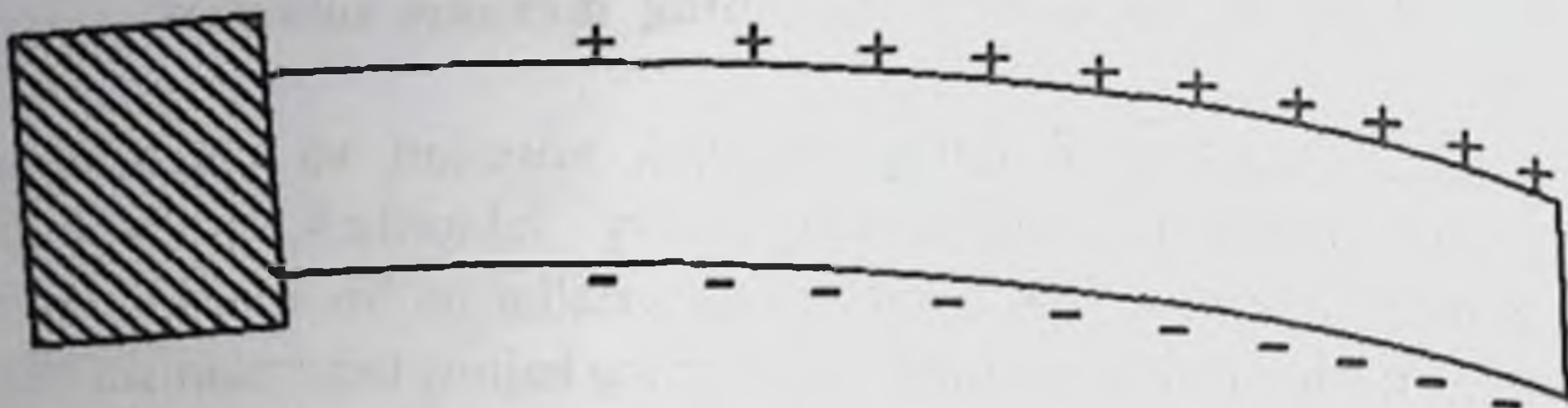
1.12-rasm. Suyak bo‘lagideformatsiyalanganda pyezoeffektning hosil bo‘lishi.
