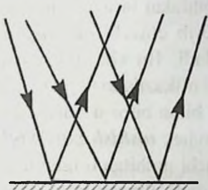
7.1-rasm. Yorug'likning tekis qaytishi
