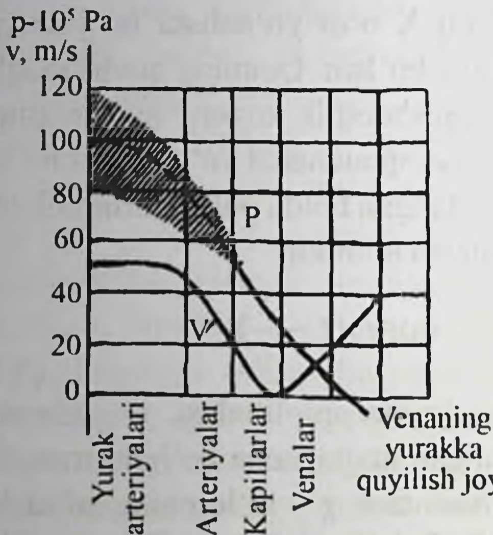
3.8-rasm. Bosimning o'rtacha qiymatining va qon oqimi tezligining qon harakatlanuvchi tomirlar turiga bog'liq holda o'zgarishini
