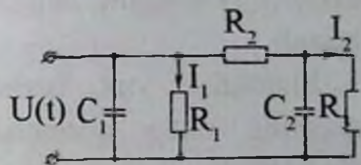
3.5-rasm. Roston modelining elektrik sxemasi
