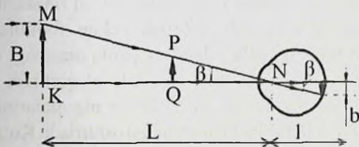
7.15-rasm. Ko'zning to'r pardasida tasvirning hosil bo'lishi
