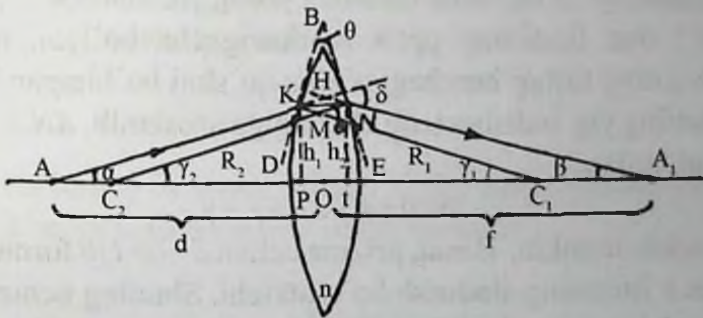
7.7-rasm. Linzada tasvir hosil qiluvchi o'qlar
