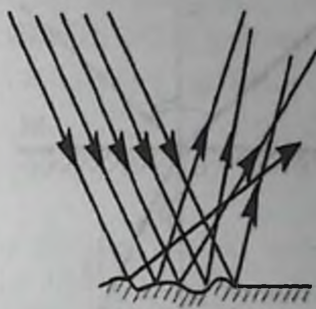
7.2-rasm. Yorug'likning tarqoq (diffuz) qaytishi
