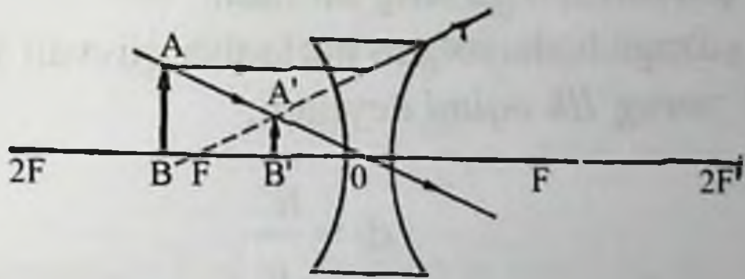
7.9-rasm. Botiq linzada tasvirning hosil bo'lishi.
