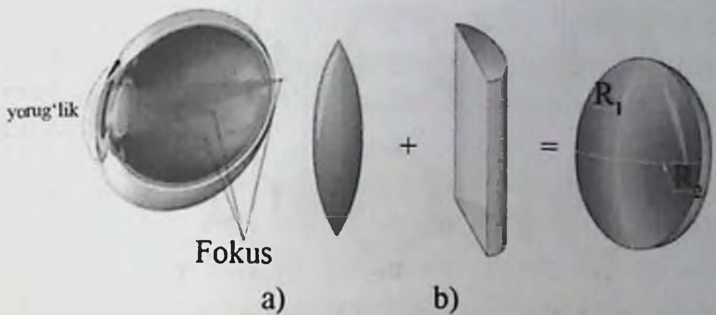
7.18-rasm. Astigmatik ko'zda tasvirning fokuslanishi (a) va uni tuzatish uchun qo'llaniladigan sferik linzalar sistemasi (b)
