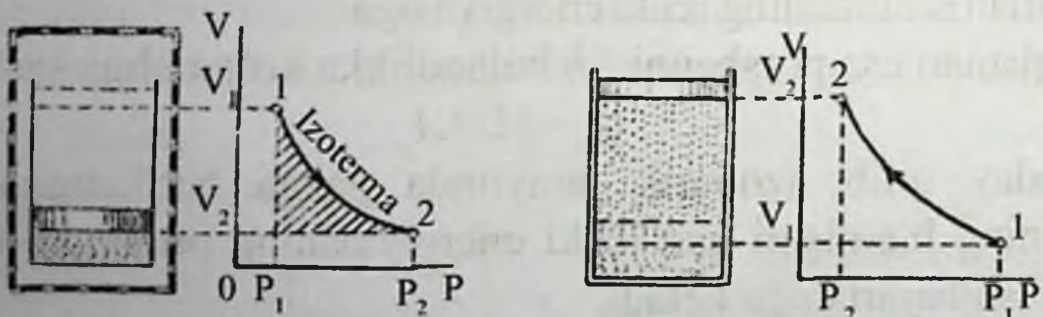
4.4-rasm. Izotermik jarayon
