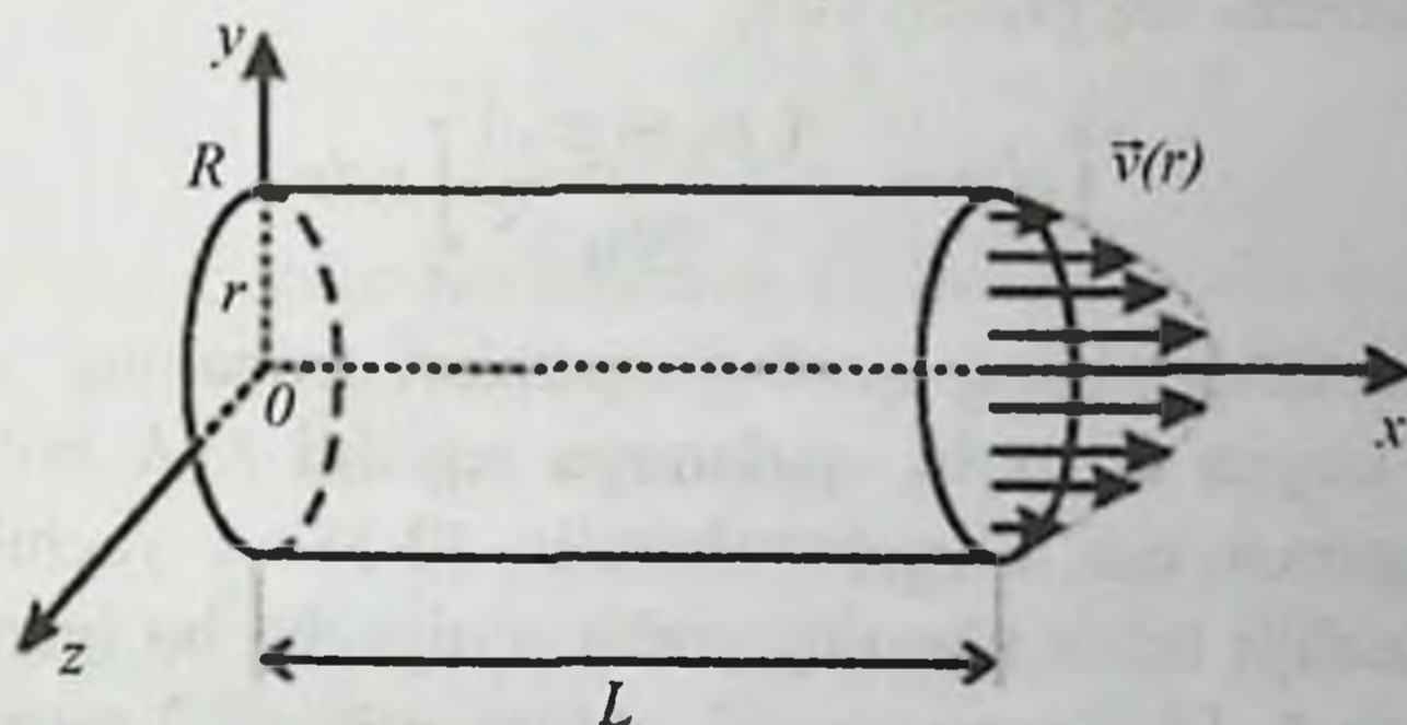
2.2-rasm. Qovushqoq suyuqlikni truba bo'ylab harakati
