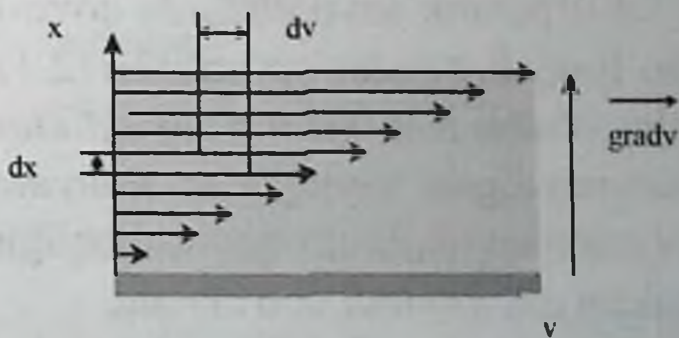
2.1-rasm. Ikki plastinka orasida qovushqoq suyuqlikning oqishi
