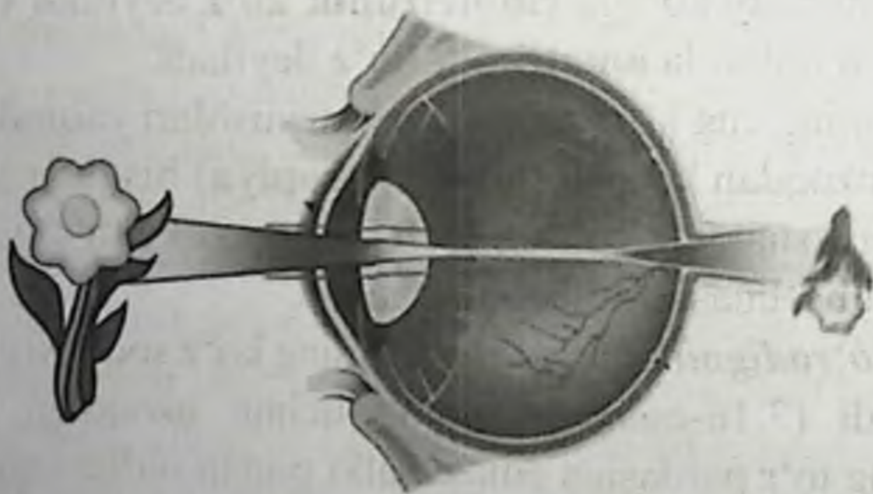
7.17-rasm. Uzoqdan ko'radigan ko'zda tasvirning hosil bo'lishi
