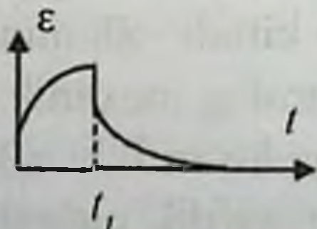
1.13-rasm. Silliqliq mushaklarning harakatini o'rganuvchi Maksvell modeli
