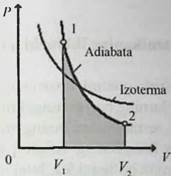
4.5-rasm. Adiabatik va izotermik kengayish
