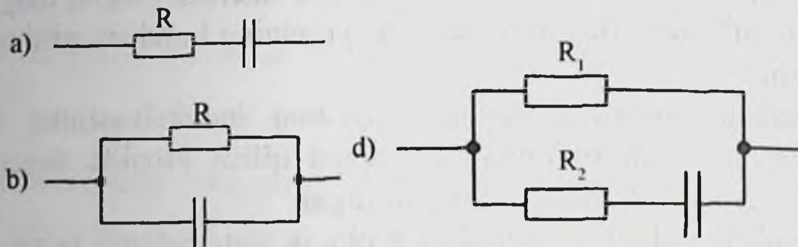
6.4-rasm. Organizm to'qimalarining ekvivalent elektrik sxemalari.
