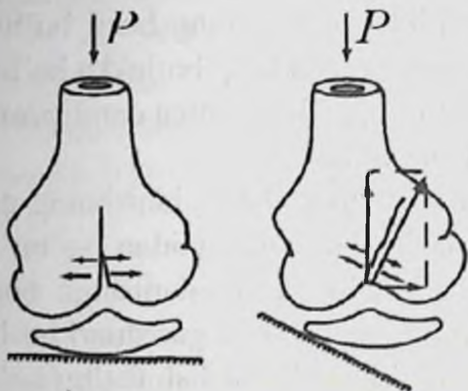
1.9-rasm. Son suyagi pastki epifizining uzilish yoki siljish deformatsiyalari ta'sirida shikastlanishi (bukilgan tizzaga yiqilganda).
