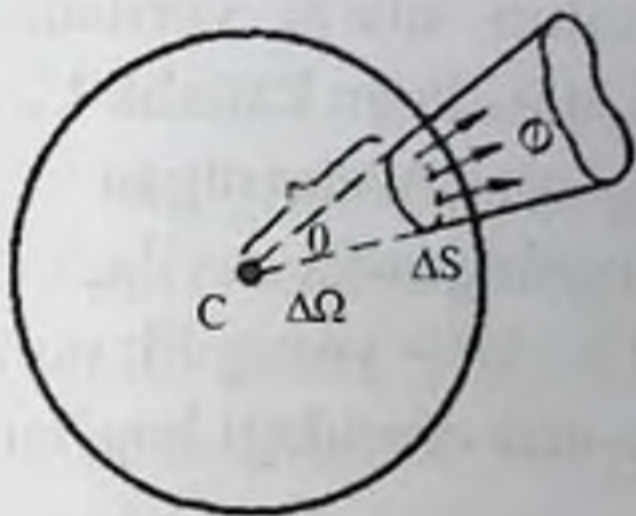
7.10-rasm. Fazoviy burchakning ifodalanishi.
