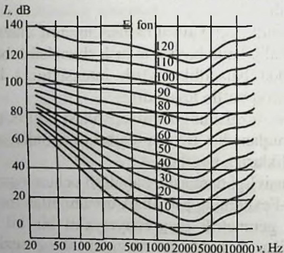
5.3-rasm. Balandlik egri chiziqlari.
