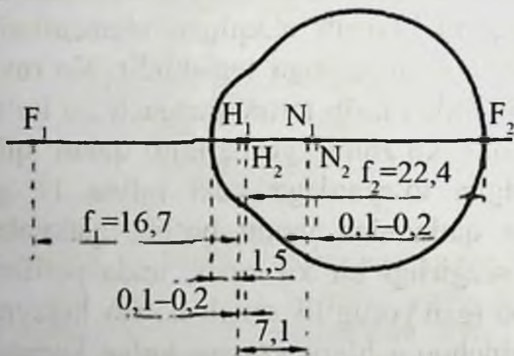
7.14-rasm. Ko'zning fokuslar, bosh nuqtalar, tekisliklar va tugun nuqtalari
