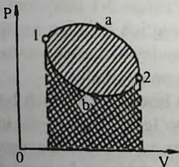
4.7-rasm. To'g'ri sikl (qaytar jarayon)
