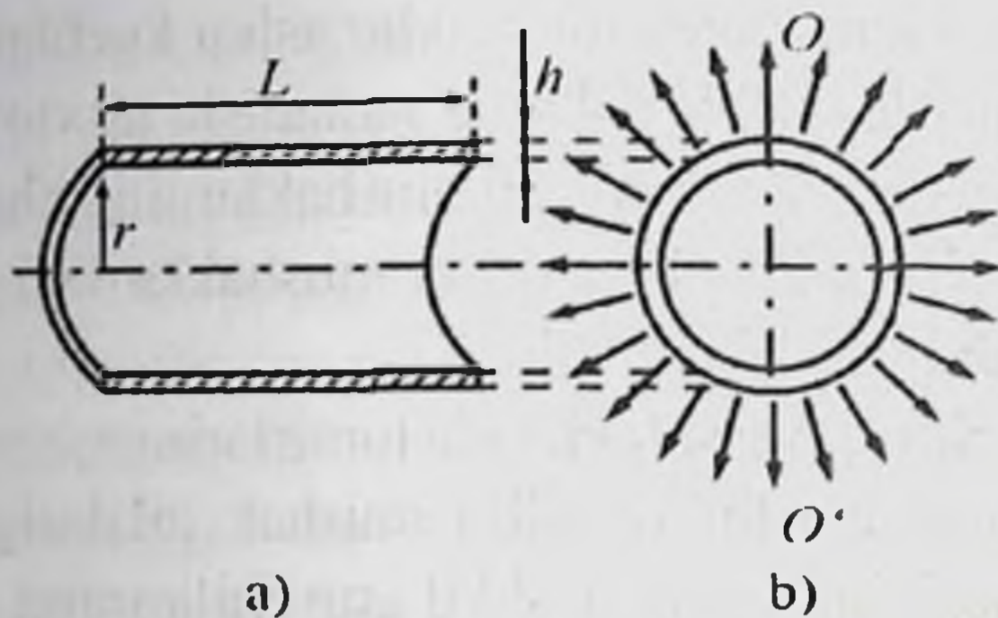
1.14-rasm. Silindrik tomirning o'q bo'ylab yo'nalgan (a) va o'qqa ko'ndalang (b) kesimlari.
