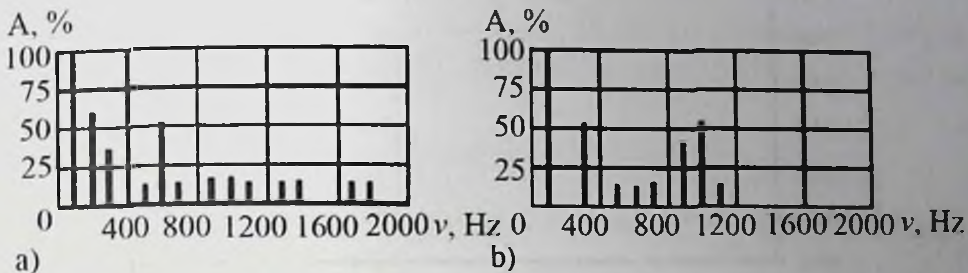
5.1-rasm. Royal'(a) va klarnet (b) notalarining spektrlari.
