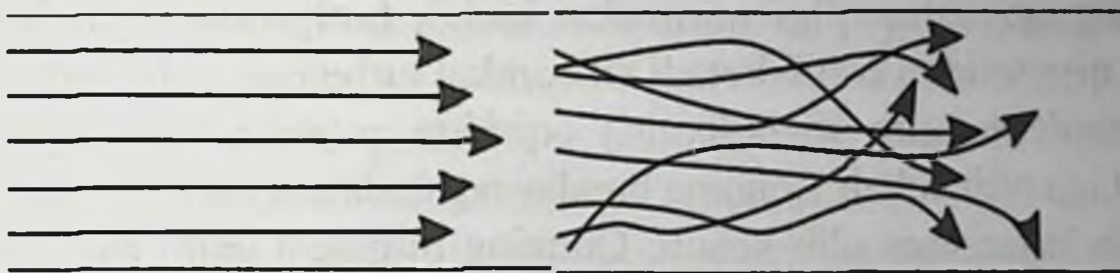
2.8-rasm. Laminar va turbulent oqimlarni sxematik tasvirlanishi.
