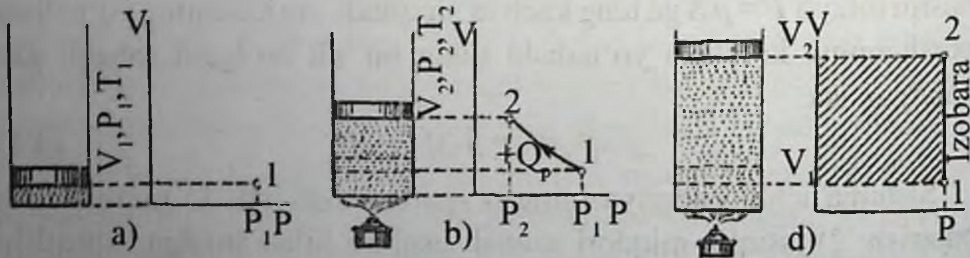
4.3-rasm. Izajarayonlar a) izoxorik jarayon b) izotermik jarayon d) izobarik jarayon
