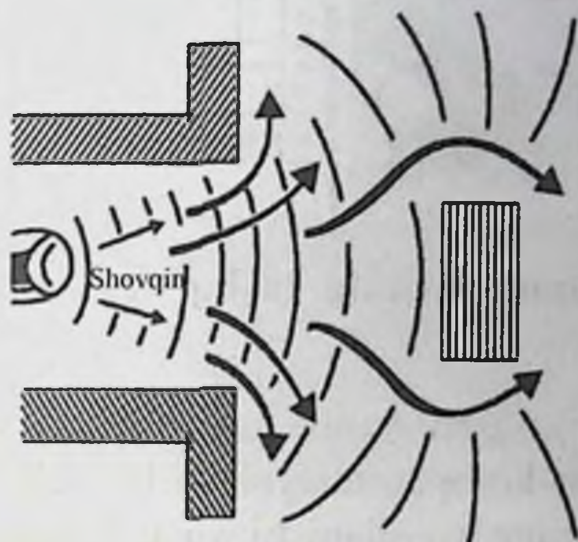
5.4-rasm. Tovush to'liqlarining difraktsiyasi.
