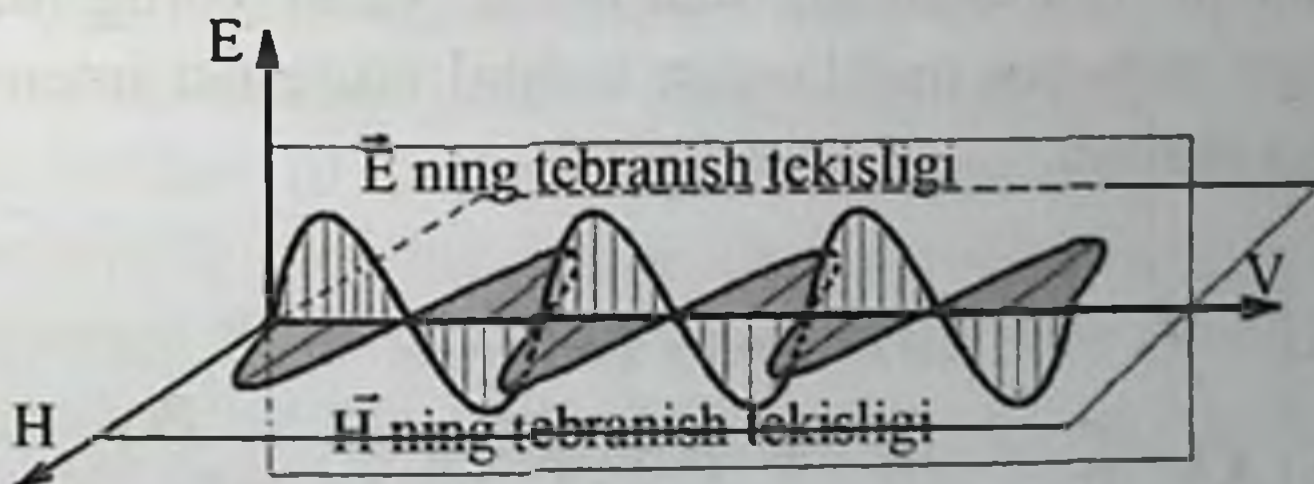
7.23-rasm. Elektromagnit to'lqinning tarqalishi ( v yo'nalishda)
