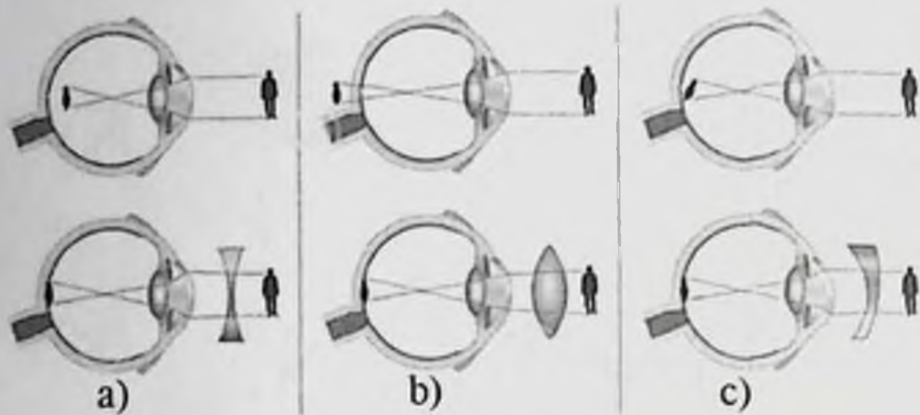
7.20-rasm. Ko'rish o'tkirligini buzilishi va uni korreksiyalash (a – yaqindan ko'rish (miopiya), b – uzoqdan ko'rish (gipermetro-piya), c – astigmatizm)
