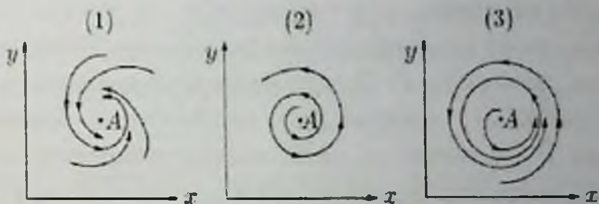
Рис. 9 Мягкая структурно устойчивая модель борьбы за существование
