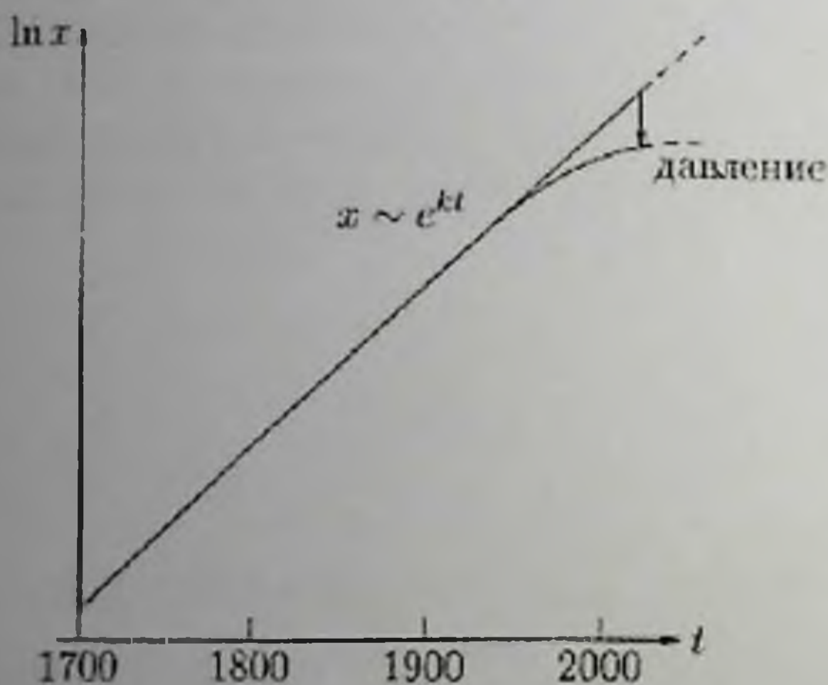
Рис. 4 Рост науки
