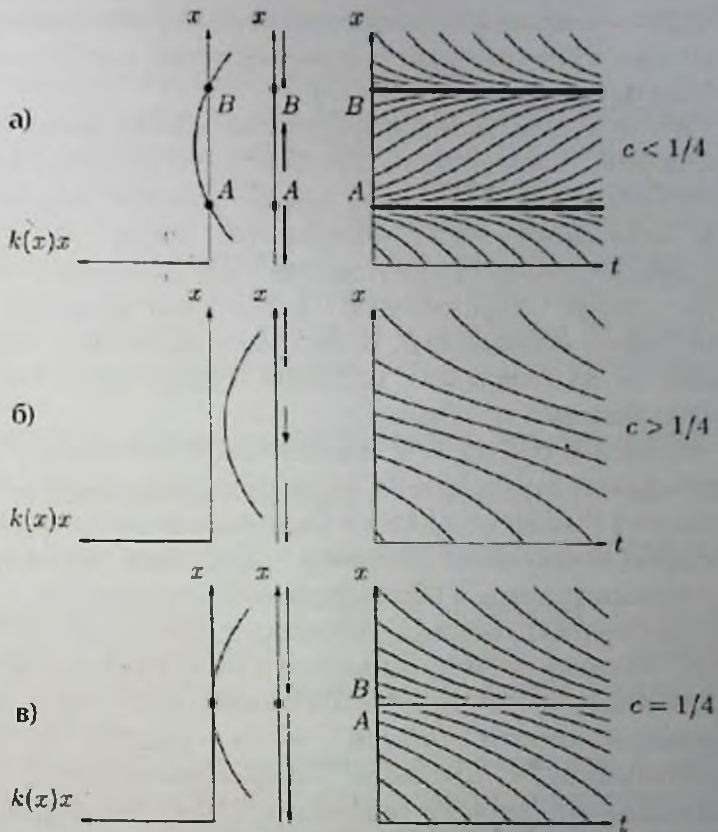
Рис. 6 Недолов (а), перелов (б) и оптимизация (в) рыболовства
