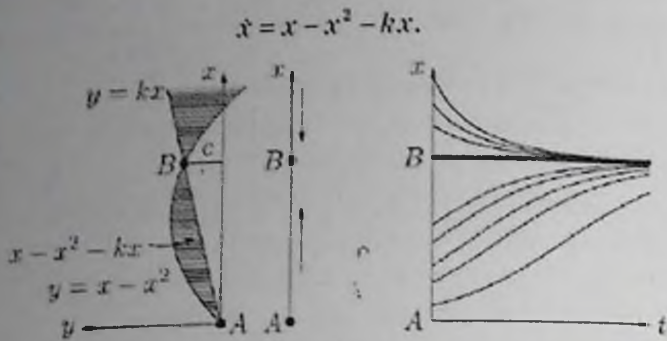
Рис. 7 Устойчивая система с обратной связью
