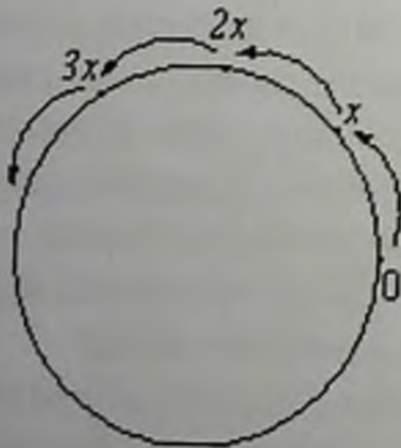
Рис. 12. К теореме Вейля.
