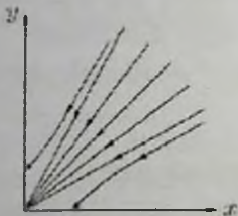
Рис. 3 Нереализуемая модель войны
