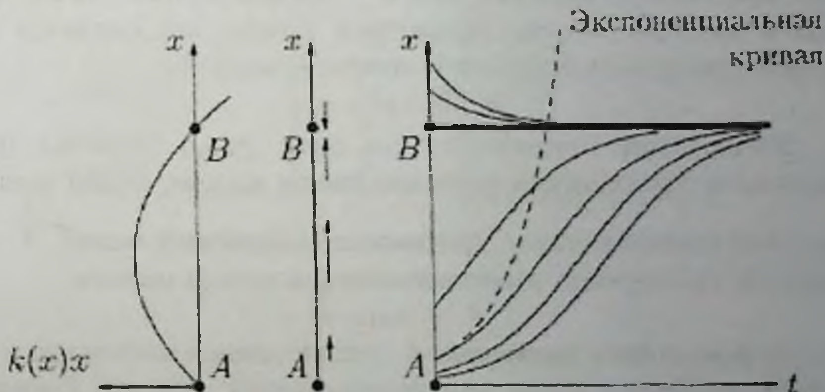
Рис. 5 Логистическая модель
