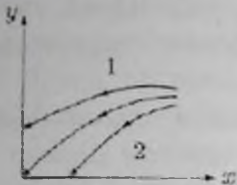
Рис. 2 Мягкая модель войны
