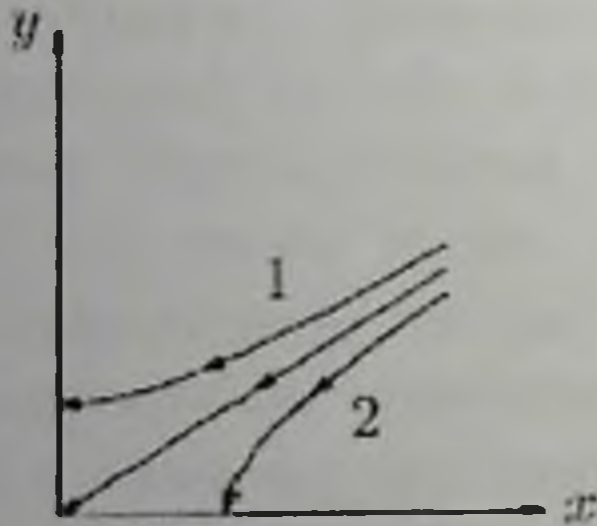
Рис. 1 Жесткая модель войны
