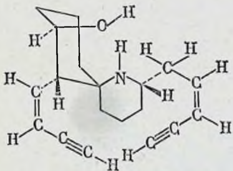
Гистрионикотоксин
