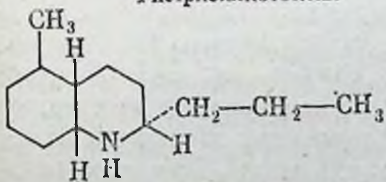
Пумилинотоксин С
