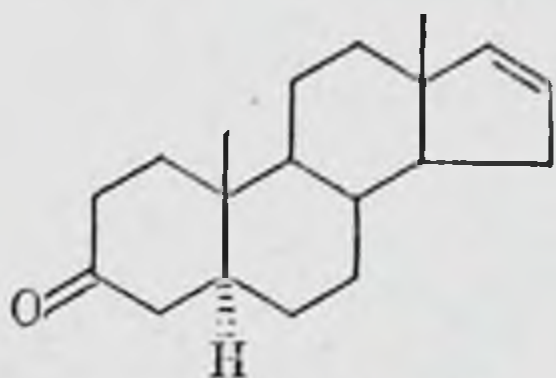
5 \alpha -андростан-16-ен-3-он
