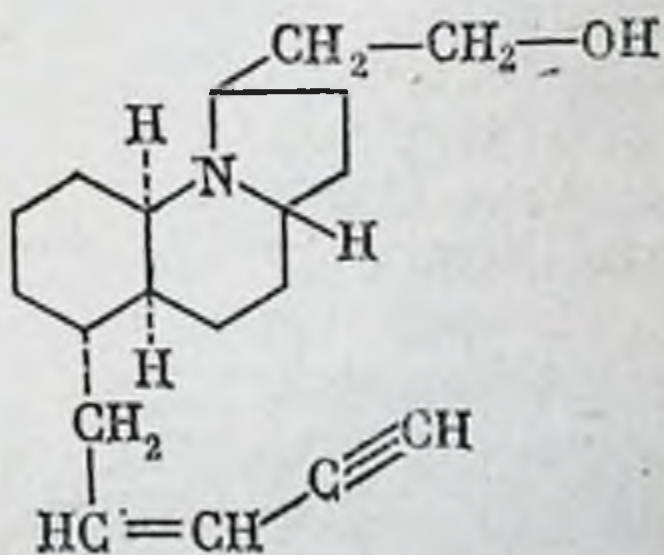
Гефиротоксин
