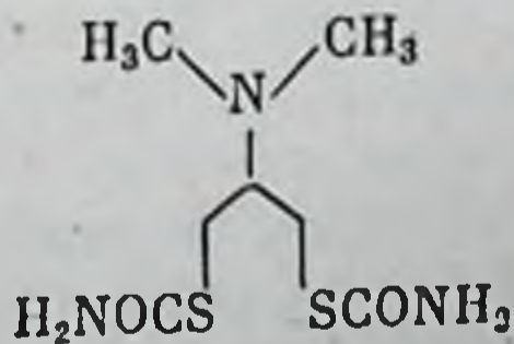
Падап
