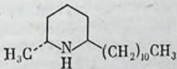
Соленопсин А
