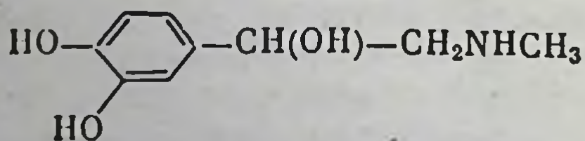
Адреналин
