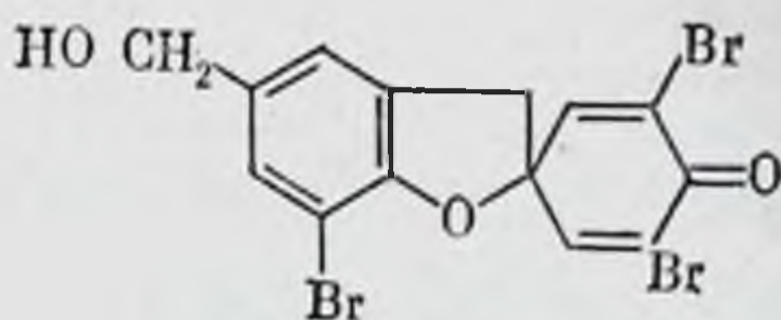
Теленин
