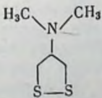
Перепстоксин
