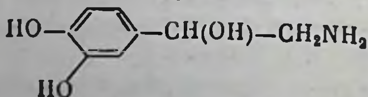
Норадреналин
