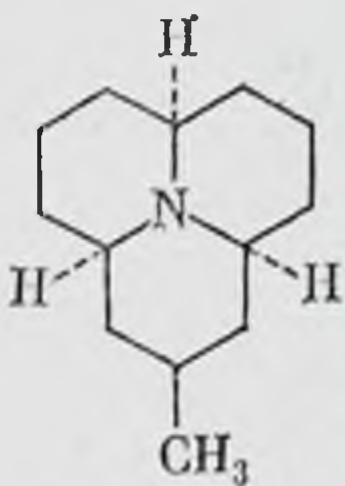
Кокцишеллин
