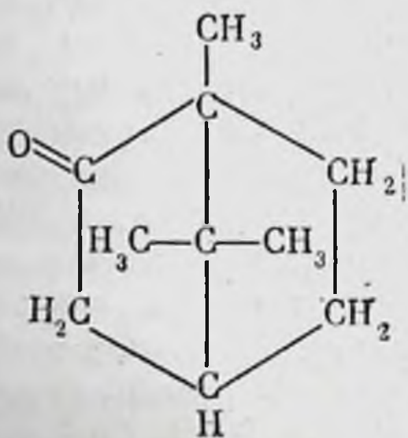
Камфора
