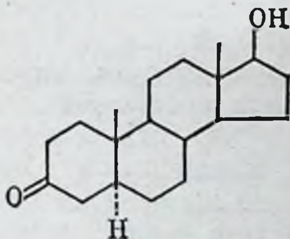
5\alpha -дигидротестостерон
