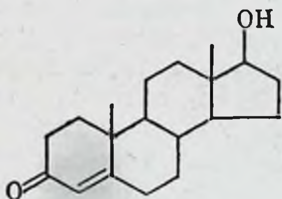
Тестостерон
