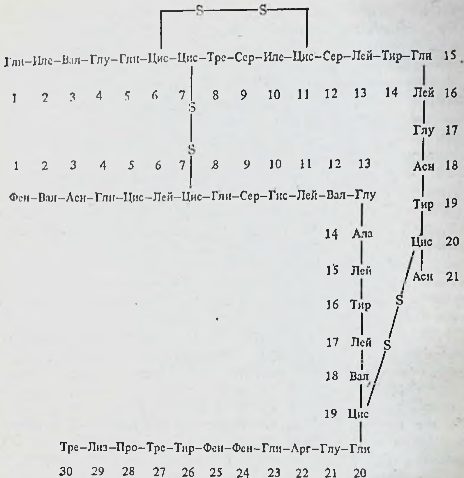
Инсулин человека
