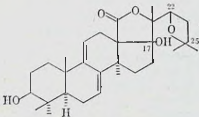
22,25-оксидоголотуриногенин
