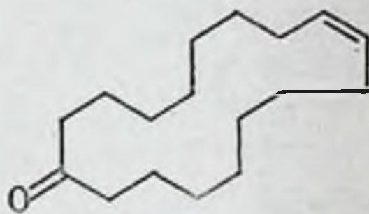
Циветон
