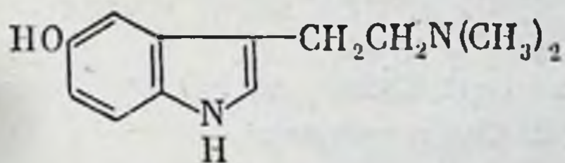
Буфотенин
