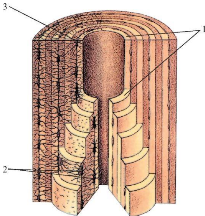
Рис. 4. Строение остеона.
