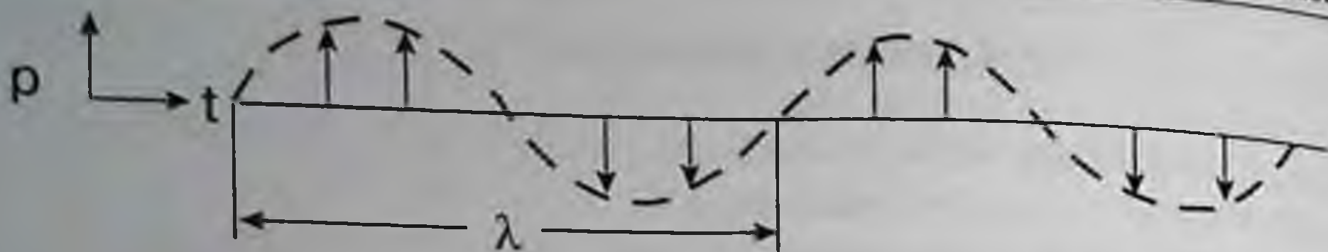
Рис. 6-19. Звуковая волна: p — звуковое давление; t — время; \lambda — длина волны
