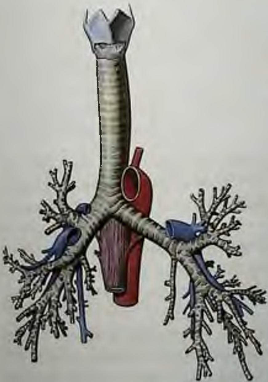
Рис. 5-6. Скелет трахеи
