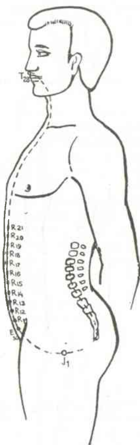
Рис. 23. Ход ИНЬ-ВЭЙ-МАЙ.
