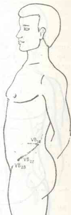
Рис. 20. Ход ДАЙ-МАЙ.
