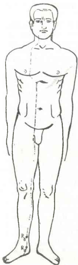
Рис. 22. Ход ИНЬ-ЦЗЯО-МАЙ.
