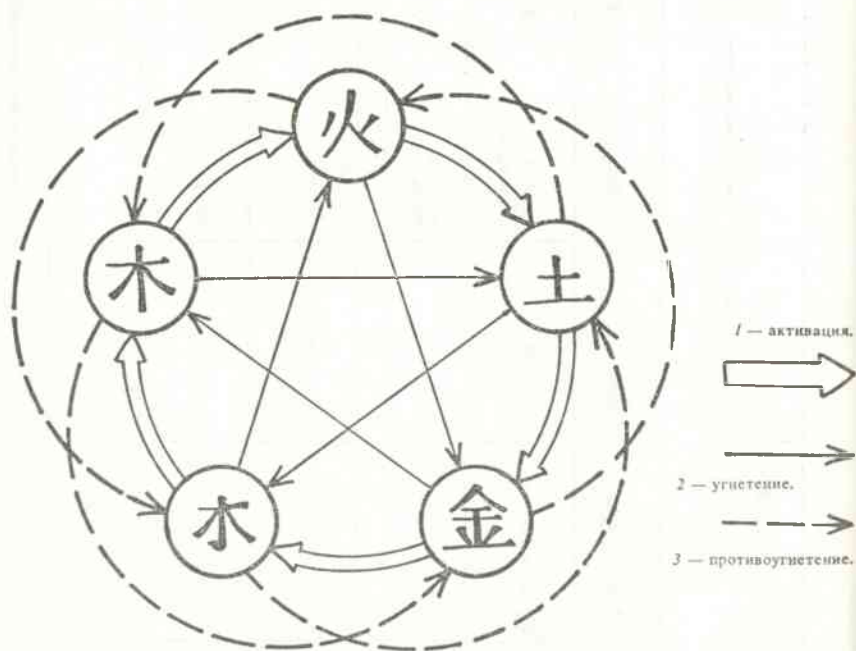
Рис. 3. Схема У-СИН.
