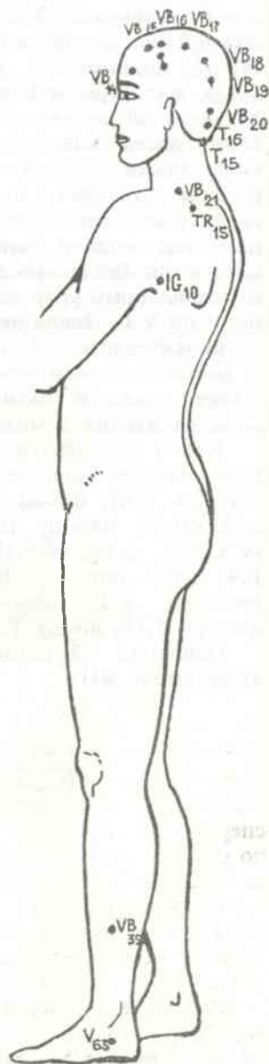
Рис. 19. Ход ЯН-ВЭЙ-МАЙ.
